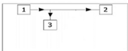
Figura.1. Schema de determinare a erorii intervalelor de intercalare în cadrele video (1 – camera video, 2 – calculator, 3 – frecvențmetru)
